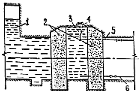
Рисунок 8 - Бетонная перемычка с контурным гидрозатвором
